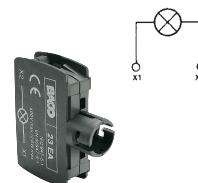
Оправка для ламп Напр. пит. лампы ≤400V, Max 2,6W
